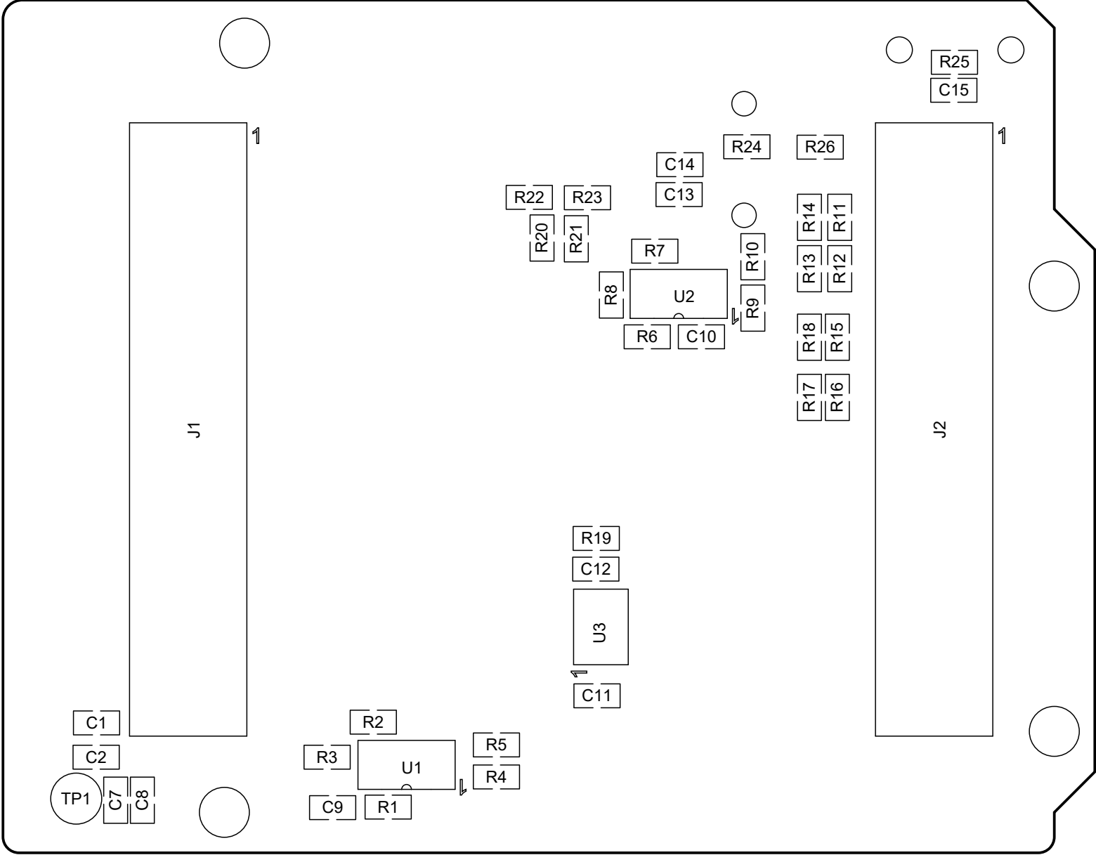
Top side (Arduino Uno Q Shield Version 2.0)
